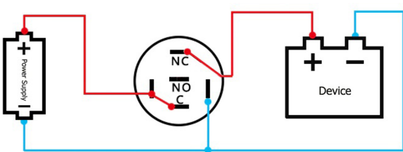
OSVETLITEV OZADJA VEDNO AKTIVNA, Kontakt - NC
