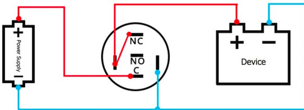
TRAJNA OSVETLITEV OZADJA, NEAKTIVNA OB PRITISKU, Kontakt - NC
