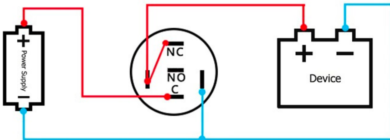
STALNA OSVETLITEV OZADJA, NEAKTIVNA PO PRITISKU, Kontakt - NC
