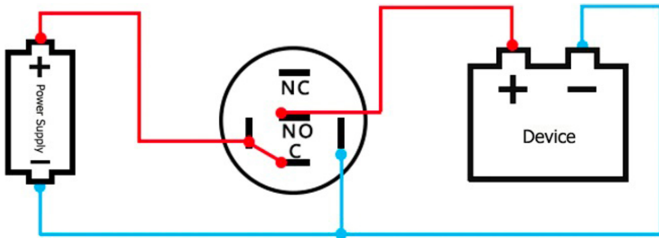
OSVETLITEV OZADJA ŠE VEDNO AKTIVNA, Kontakt - NE
