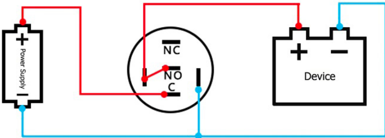
HINTERGRUNDBELEUCHTUNG INAKTIV, AKTIV NACH DRÜCKEN, Kontakt - NEIN
